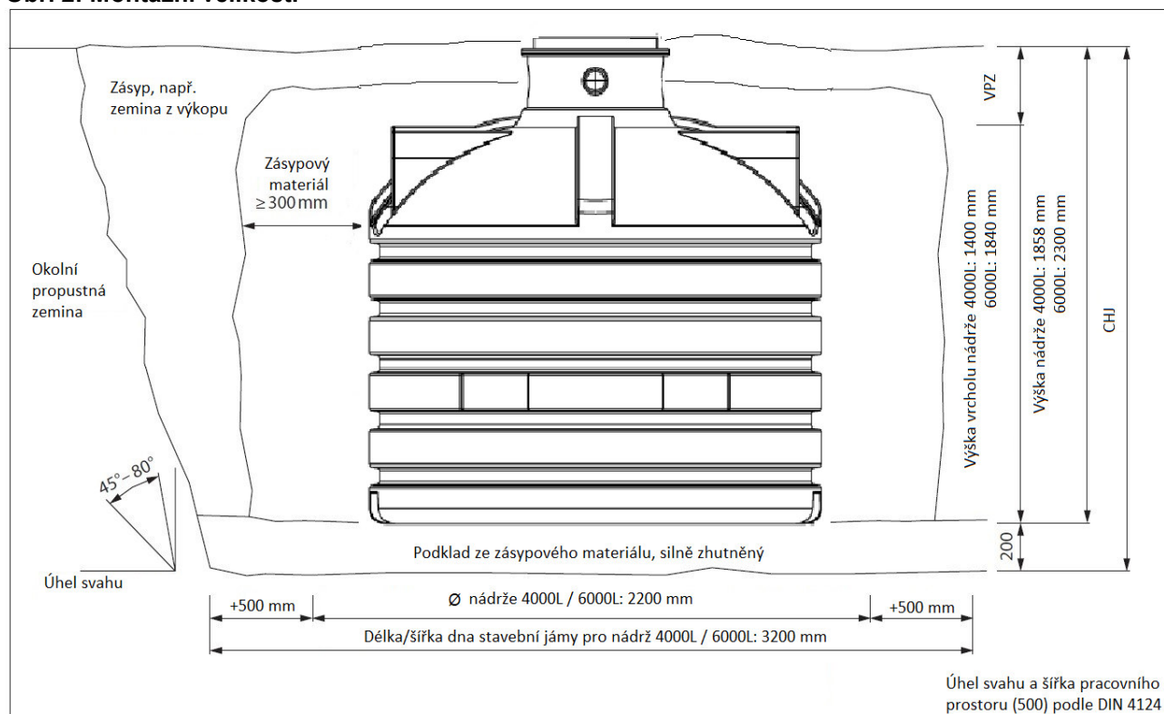
Obr. 2: Montážní velikosti
