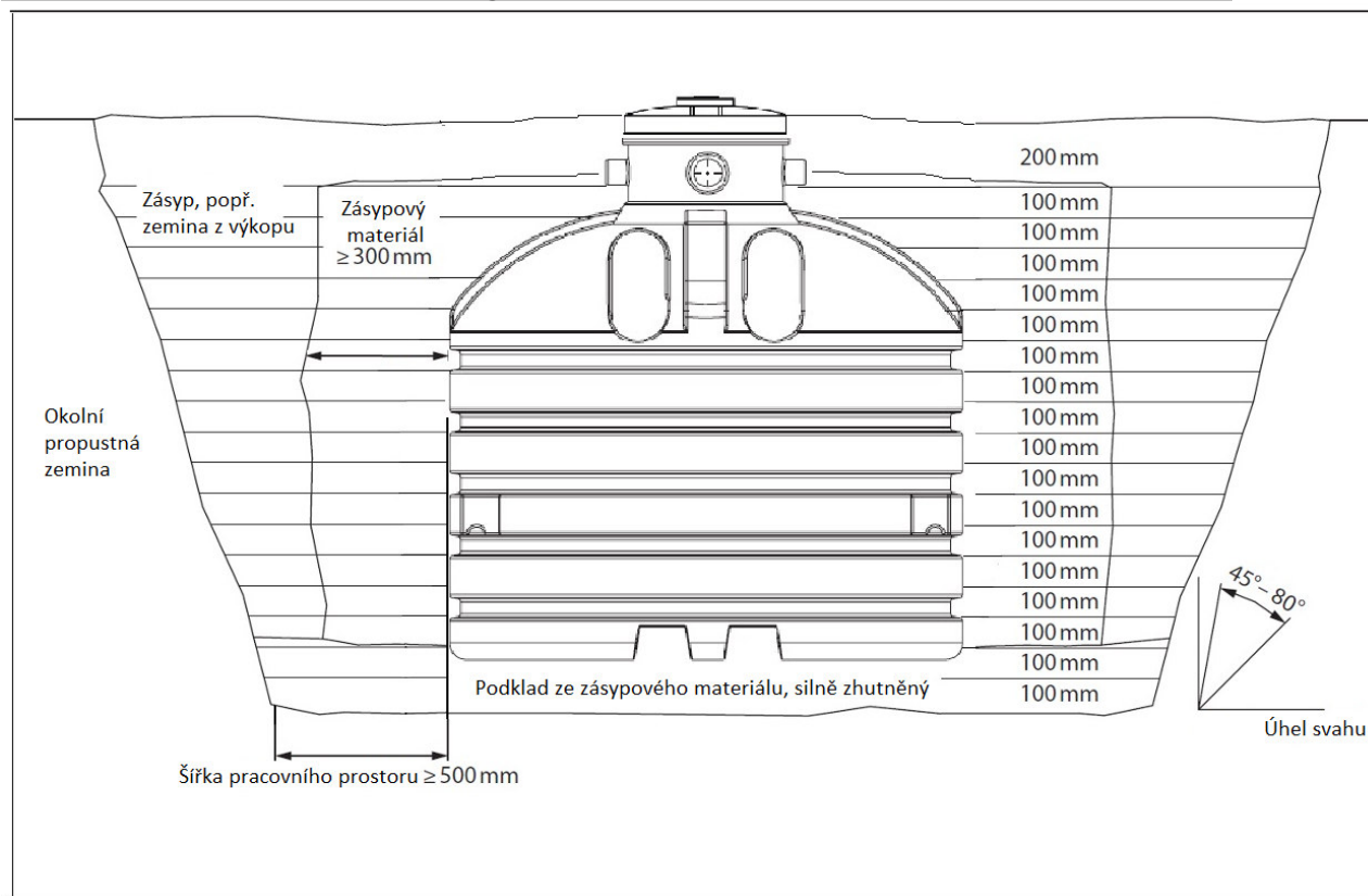
Obr. 4: Provedení montáže na příkladu podzemní nádrže Oasis 6000 litrů s poklopem nádrže Basic
